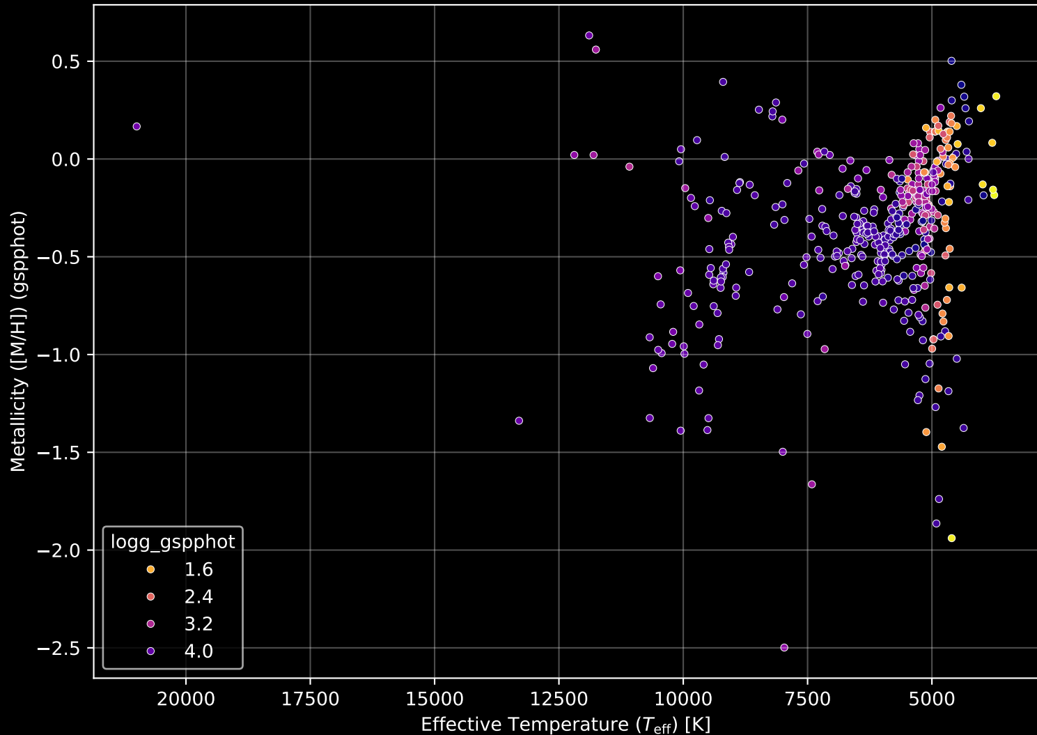
APOGEE DR17 Field: [M35N2158_btx] Stellar Population Parameters (n= 453)
